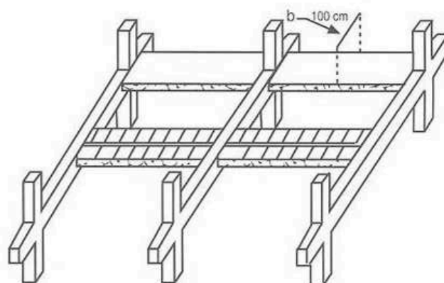
Fig 2 - Modello pratico costruttivo dello stesso schema di figura 1 ad orditura unidirezionale su un'ossatura portante in c.a..
